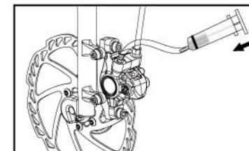
f-6. Behälter durch Hineindrücken des Spritzenkolbens befüllen
